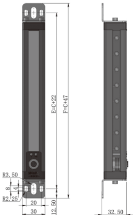
取料光栅带安装支架尺寸
